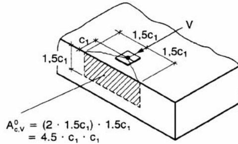
图4.4.2-1 单锚栓混凝土理想破坏楔形体定义 [4]
