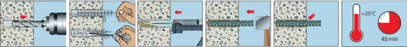
安装示意图
