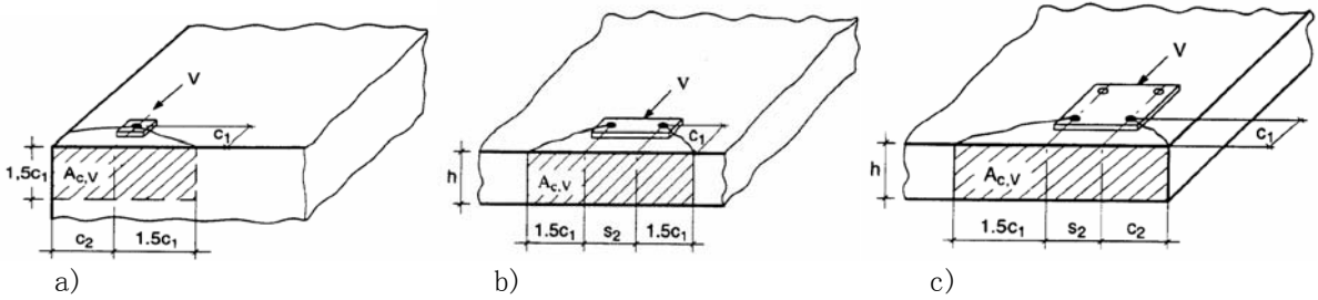
图4.4.2-2 实际破坏楔体在侧向的投影面面积计算举例 [4]
