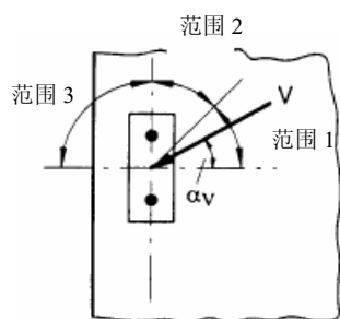
图4.4.2-3 夹角定义[4]
