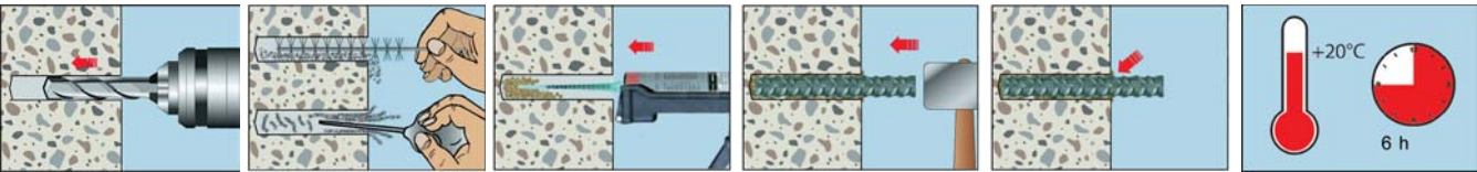
安装示意图
