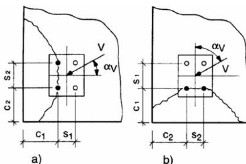
图4.4.2-4 锚基角边受剪，双边缘验算举例[4]
