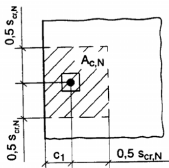
图4.3.3-2 近边缘单锚[4]
