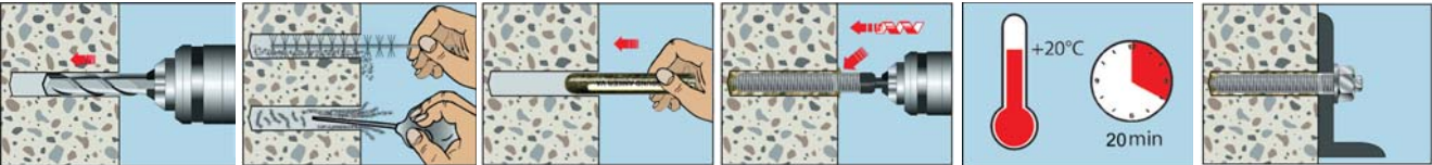
安装示意图
